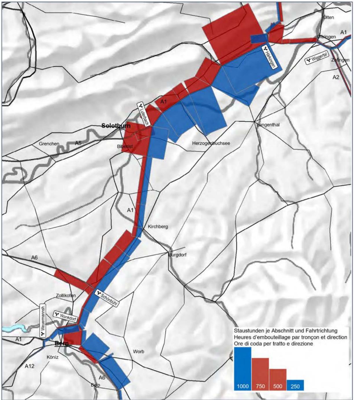
Abbildung 37: Staustunden 2022 auf den Nationalstrassen in der Region Bern / Solothurn Quellen: ASTRA: VMON, Viasuisse
