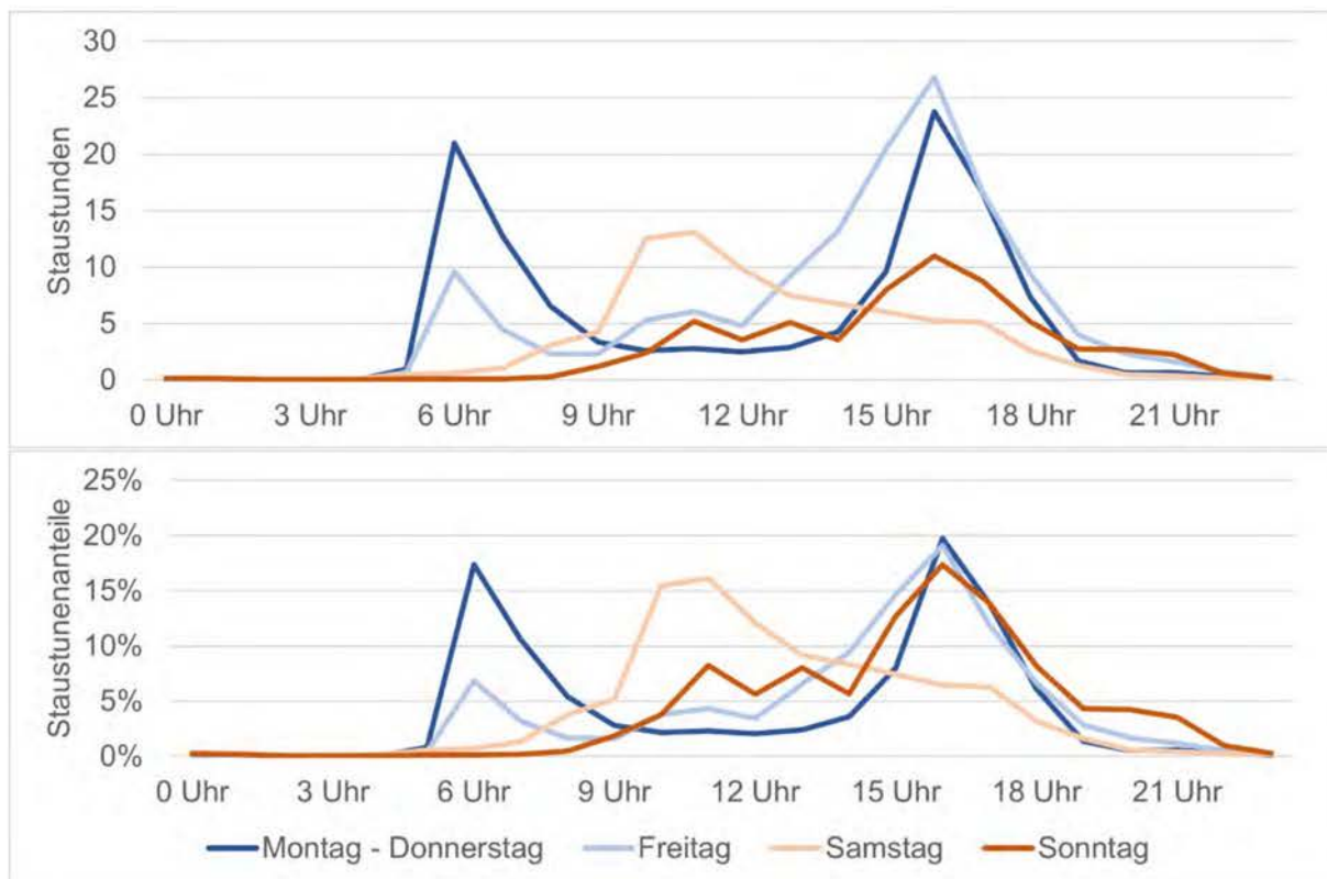
Abbildung 50: Staustunden und Staustundenanteile 2022 auf den Nationalstrassen im Tagesgang nach Tagestyp Quellen: ASTRA: VMON, Viasuisse
