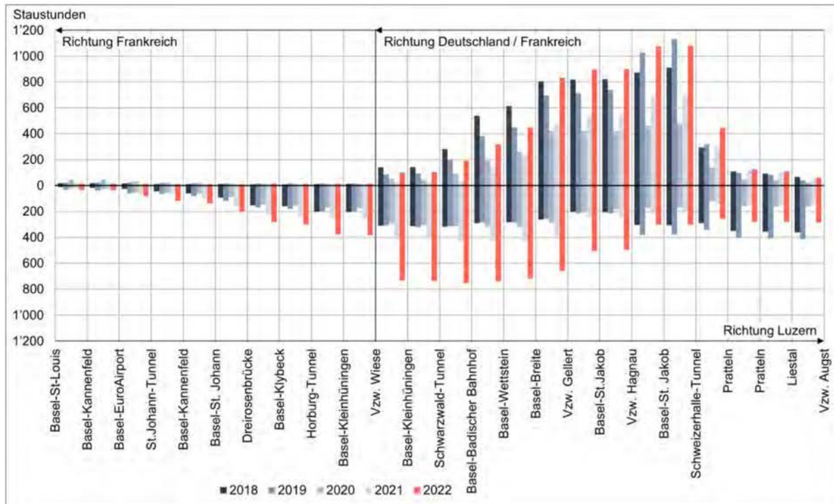
Abbildung 34: Entwicklung der Stautunden auf der A2/A3 zwischen Basel und Augst Quellen: ASTRA: VMON, Viasuisse
