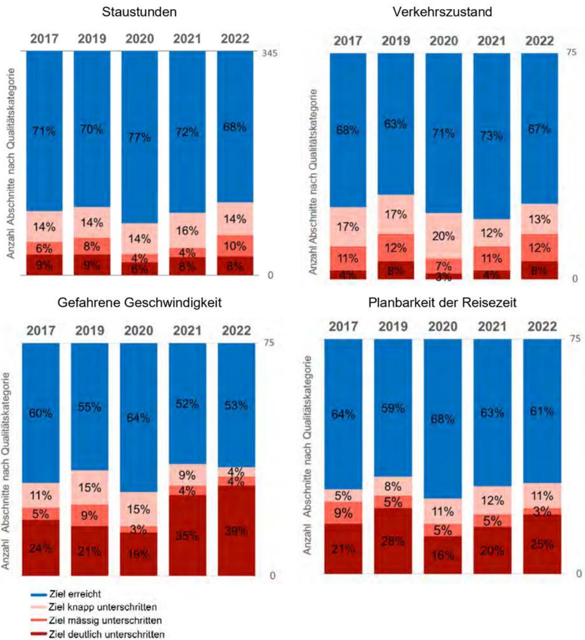
Abbildung 58: Entwicklung Angebotsqualität der Indikatoren «Stautunden», «Verkehrszustand», «Gefahrenere Geschwindigkeit» und «Planbarkeit der Reisezeit».
